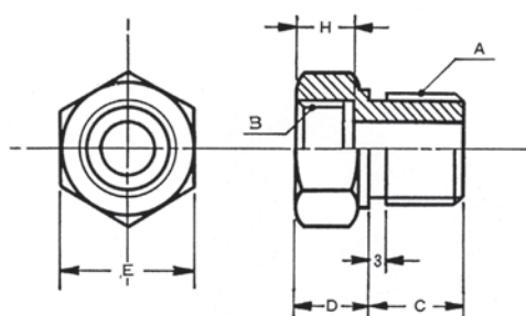
ストレートユニオン Straight union
