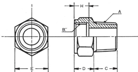
テーパユニオン Taper union
