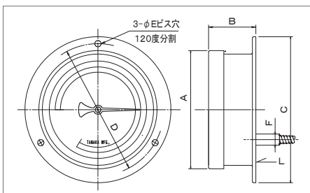
BR・BN-MH 形共通寸法図
