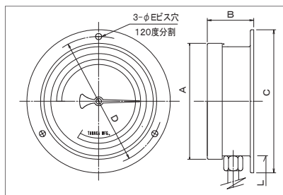
BN-MG 形共通寸法図
