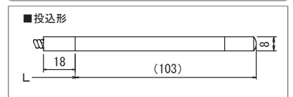
全機種共通 標準感温部寸法図
